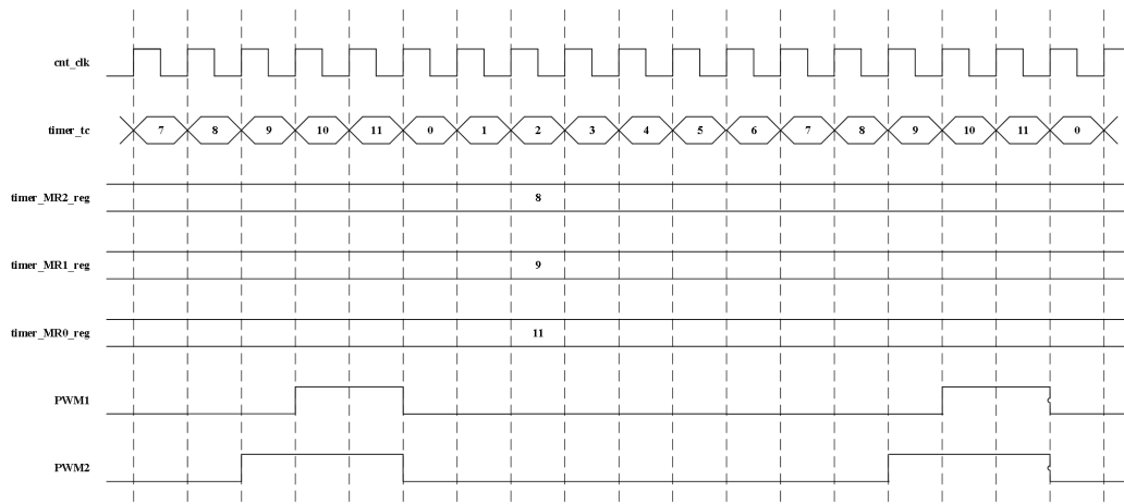
图 12-20 PWM 模式为 010 输出波形（递增）
