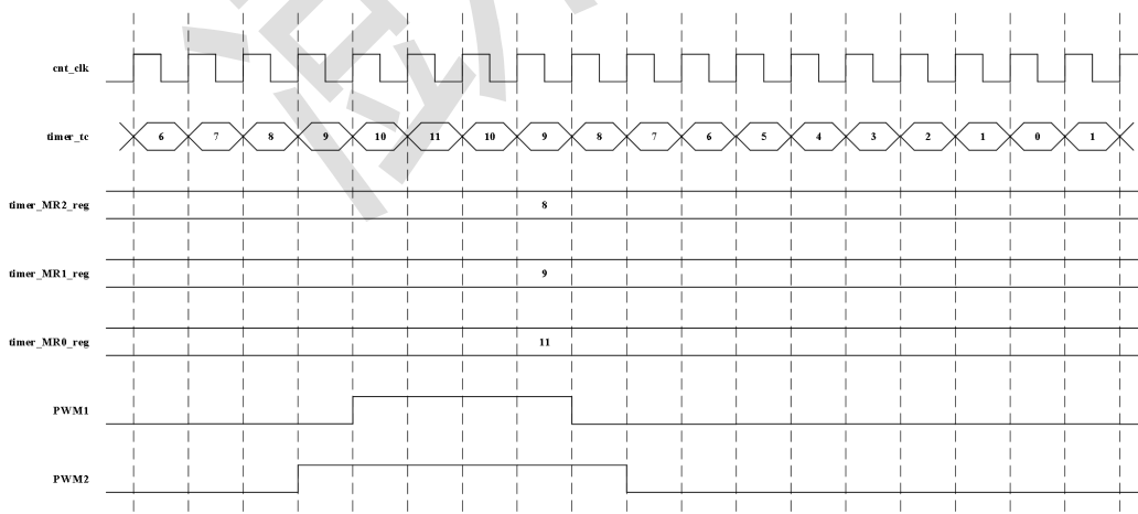
图 12-22 PWM 模式为 010 输出波形（交替）
