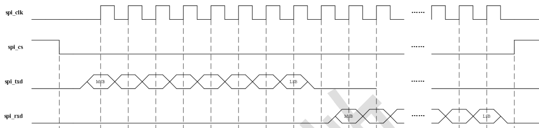
图 21-2 National Microwire 模式单帧数据传输时序图
