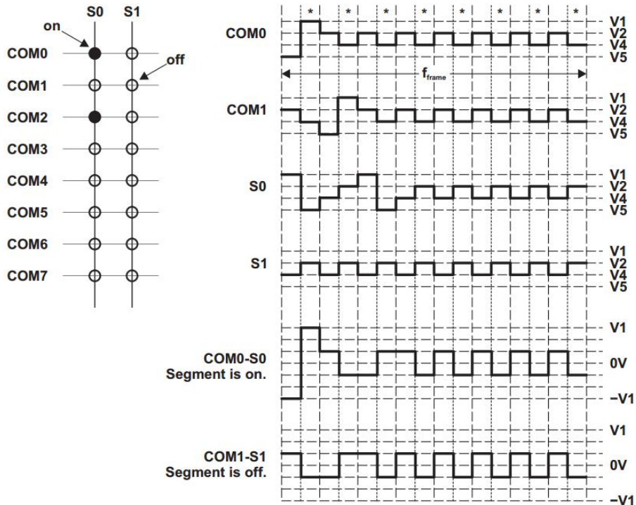
图 16-6 8COM, 1/3 偏压下的 TypeA 波形
