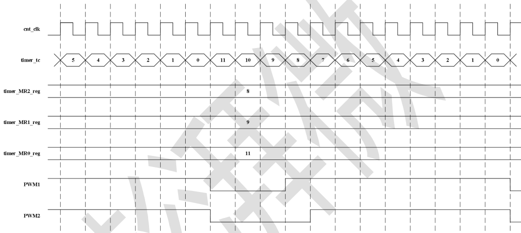
图 12-18 PWM 模式为 001 输出波形（递减）
