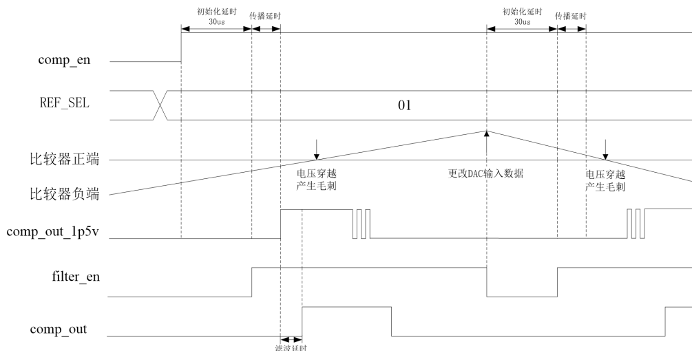
图 25-3 比较器比较控制时序 (REF=01)
