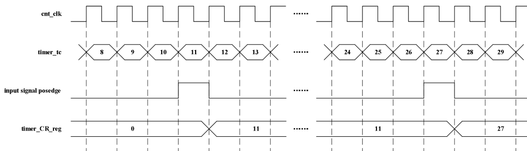
图 12-15 TMRn_TC 值被存入 TMRn_CR 寄存器且 TMRn_TC 不复位（仅捕捉上升沿） 软件可通过配置 TMRn_CCR 寄存器来选择 TMRn_TC 在捕捉通道信号跳变后 TMRn_TC 是复位重新开始计数（图 12-14）还是继续计数（图 12-15）。
