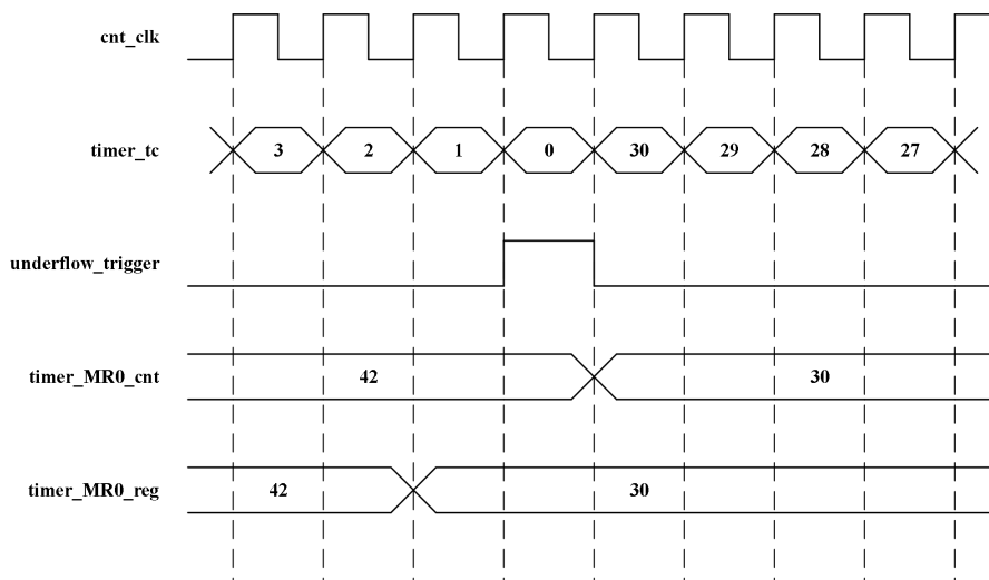
图 12-8 递减计数时自动更新匹配值
