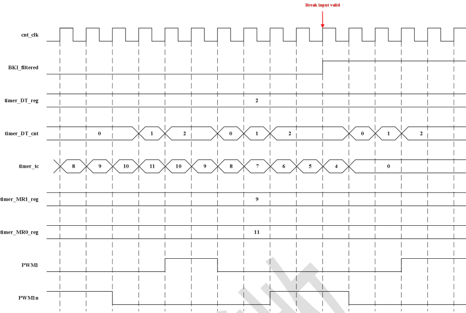
图 10-23 刹车输入有效电平时，死区插入的互补 PWM 输出波形 (PWM1 = 1)
