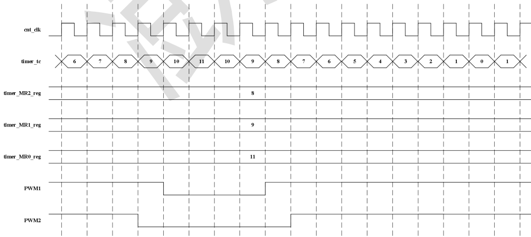
图 12-19 PWM 模式为 001 输出波形（交替）
