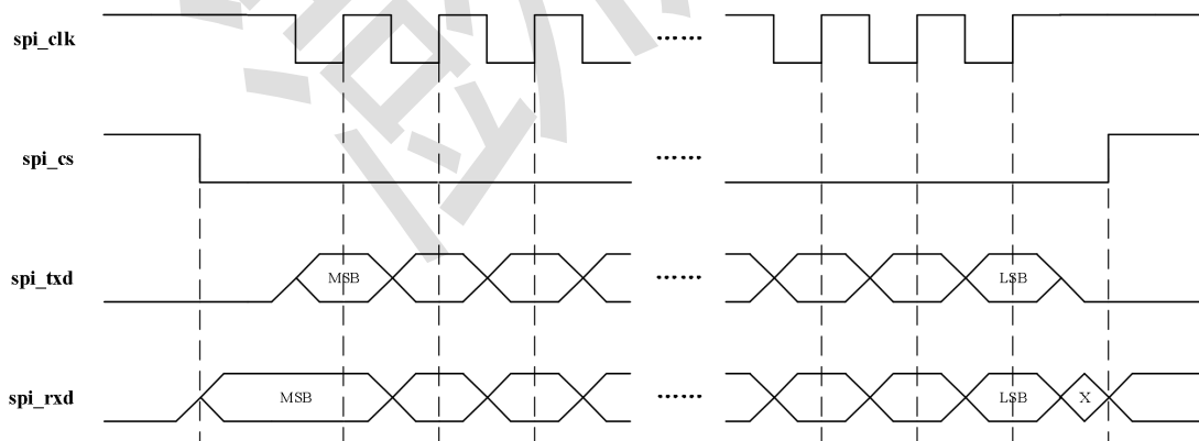
图 21-7: 模式 11 时序图 (SCLKP=11)
