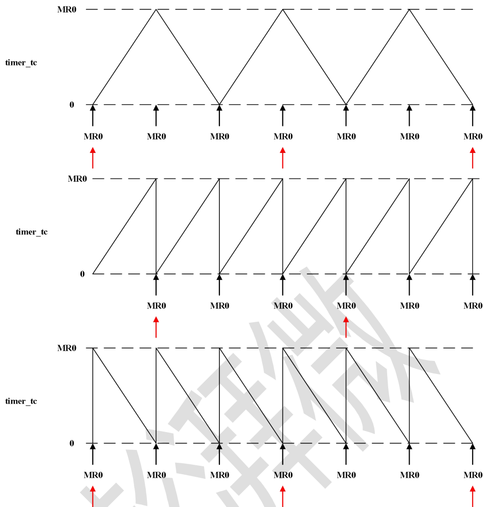
图 12-5 累计溢出输出中断示意图 (INT_RPT = 2)
