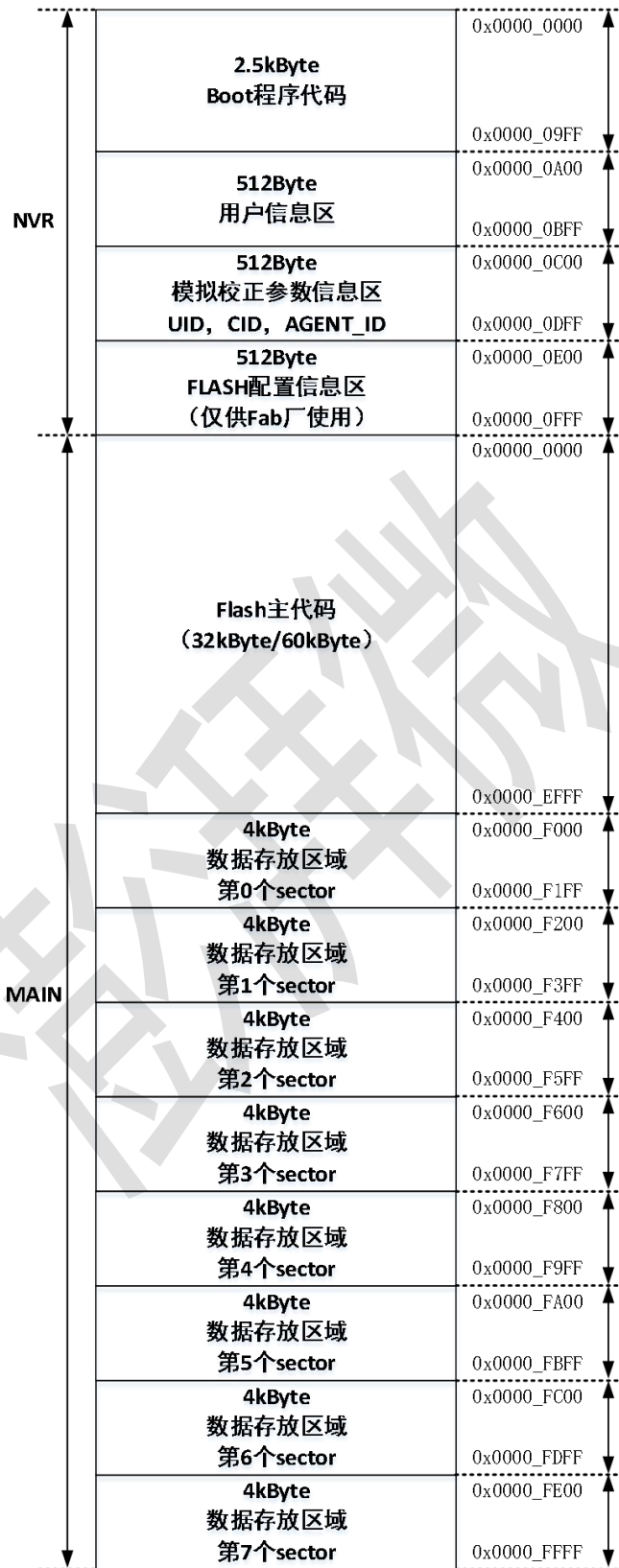
图 28-1 64KByte Flash 规格芯片的 Flash 区域划分 (地址单位: Byte)
