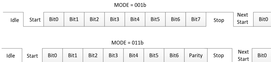
图 20-2: UART 8 位数据帧格式 (普通极性)
