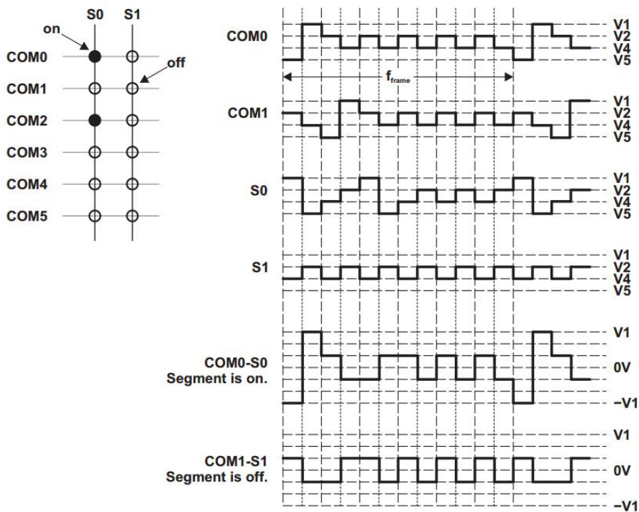
图 16-5 6-COM, 1/3 偏压下的 TypeA 波形
