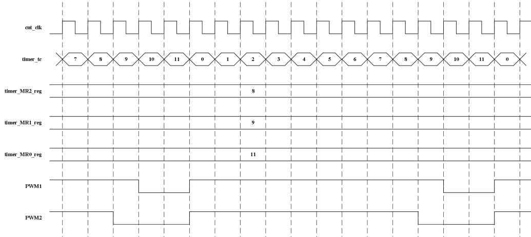
图 12-17 PWM 模式为 001 输出波形（递增）
