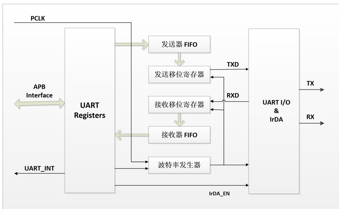
图 20-1: UART 框图
