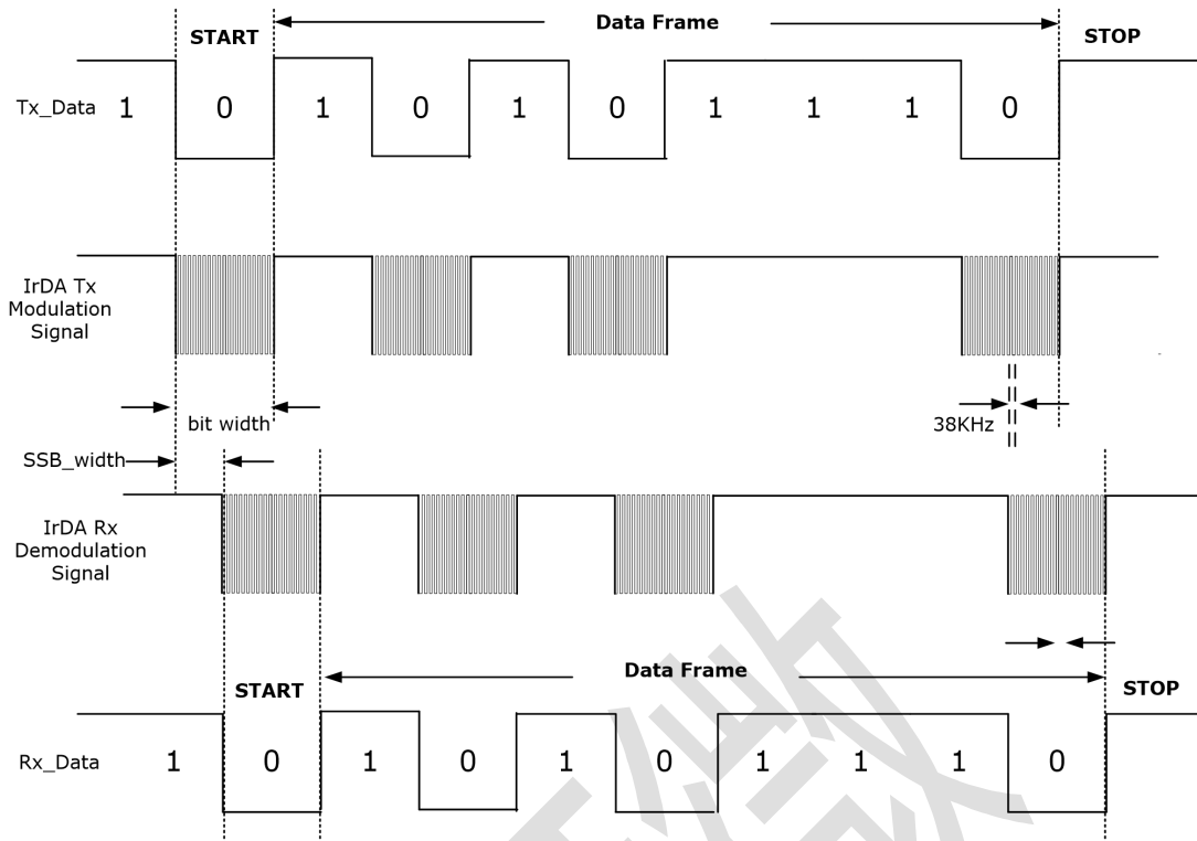
图 20-6: IrDA 调制与解调(普通极性)
