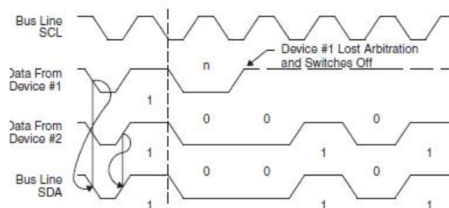
图 22-2 I 2 C 两个主机仲裁过程示意图
