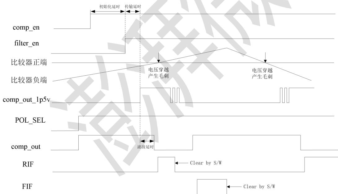
图25-5. 比较器状态更新时序图（REF=00/10）
