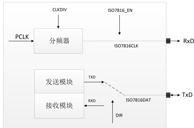
图 20-7: UART ISO7816 模块功能示意图
