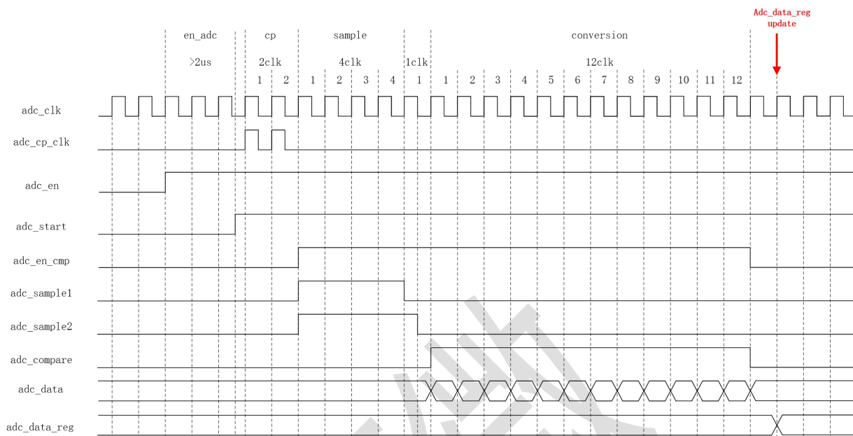
图23-1 单次转换时序
