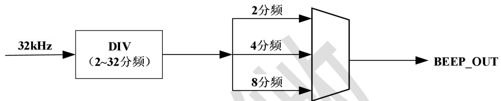
图 19-1 蜂鸣器工作原理图
