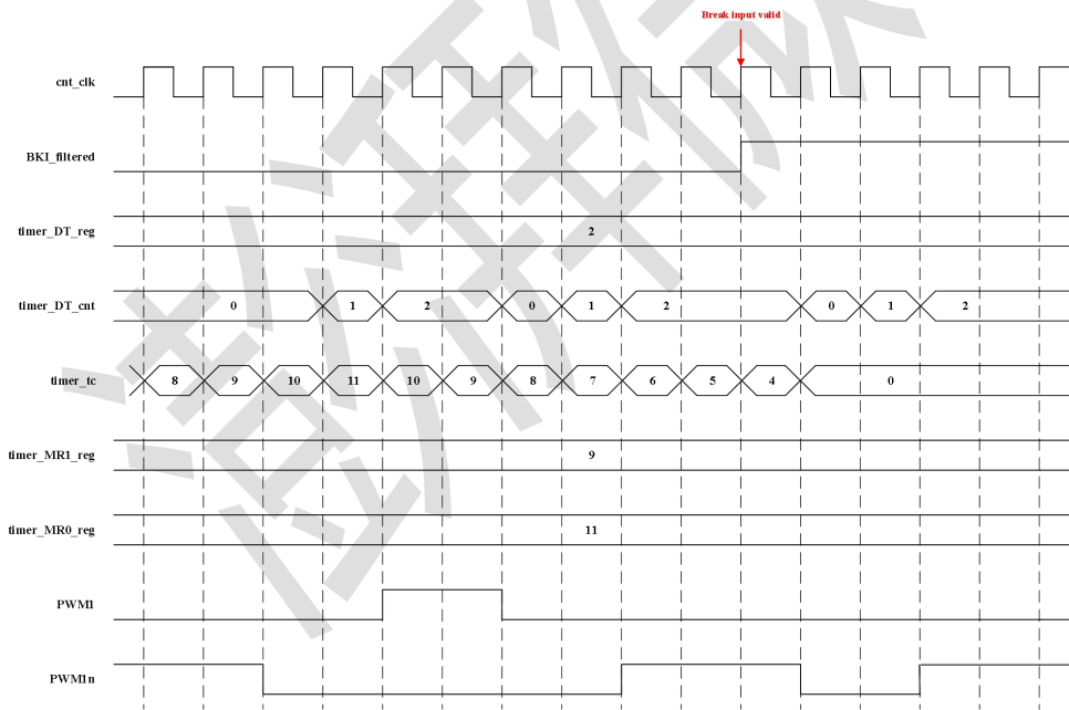
图 10-23 刹车输入有效电平时，死区插入的互补 PWM 输出波形 (PWM1 = 0)
