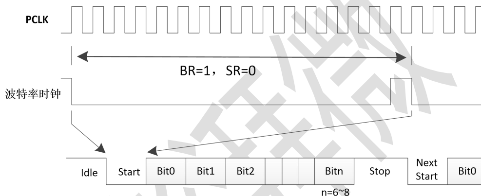
图 20-4: UART 时钟和数据帧时序
