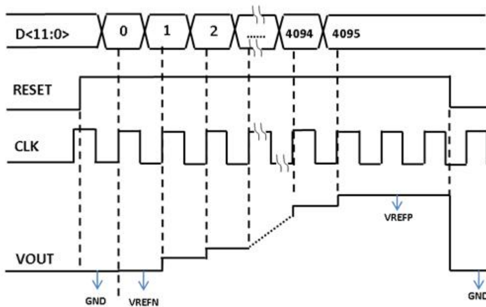
图 24-2 DAC 转换时序图
