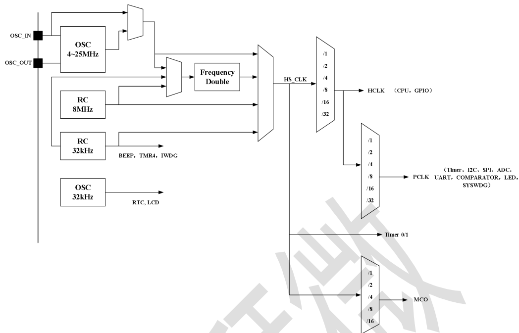
图 8-1 时钟结构图
