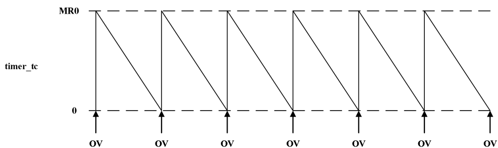
图 13-3 递减计数示意图
