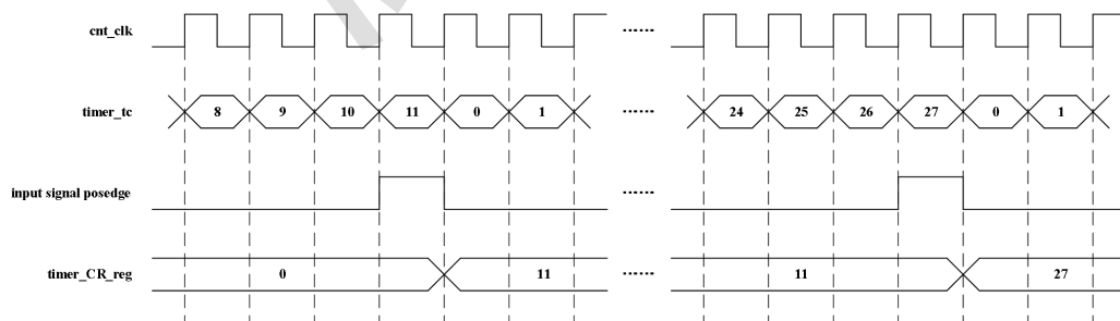
图 12-14 TMRn_TC 值被存入 TMRn_CR 寄存器且 TMRn_TC 复位（仅捕捉上升沿）
