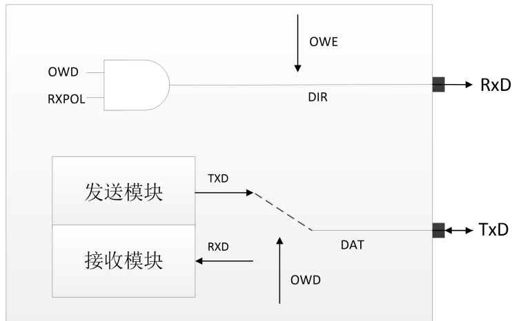
图 20-9: UART 单线半双工通讯模式功能示意图
