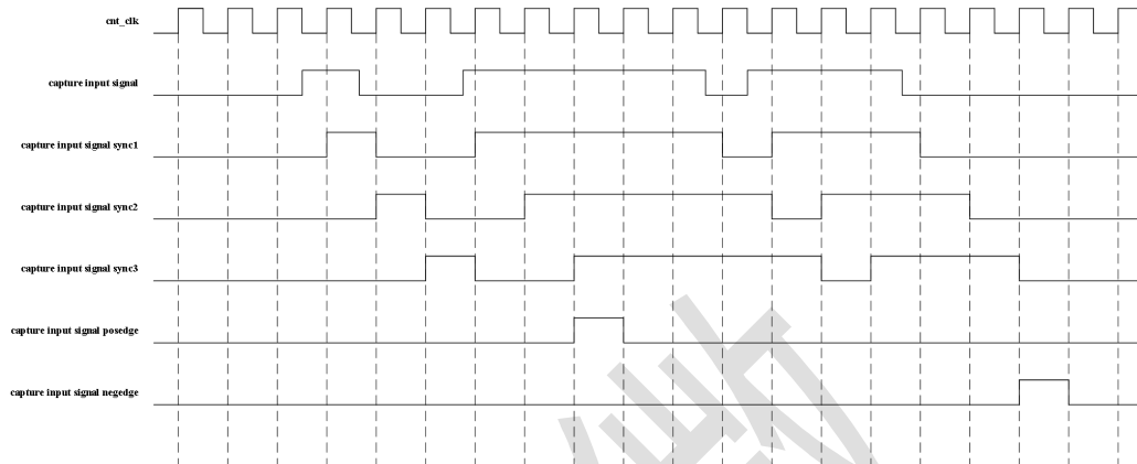
图 12-13 捕捉通道信号同步滤波
