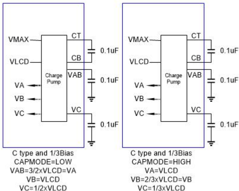
图 16-1 C 型 LCD 偏置电压
