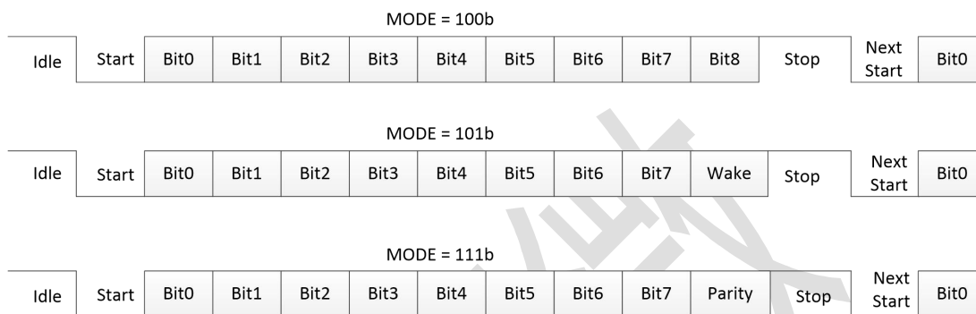
图 20-3: UART 9 位数据帧格式 (普通极性)
