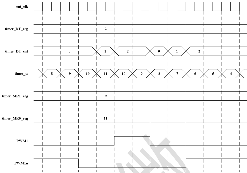
图 12-24 死区插入的互补 PWM 输出波形
