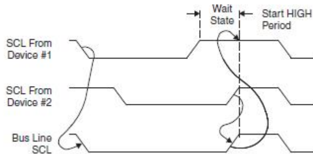
图 22-3 I 2 C 总线仲裁过程中 SCL 波形示意图
