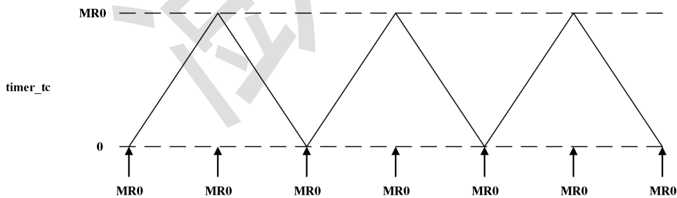
图 12-4 交替计数示意图
