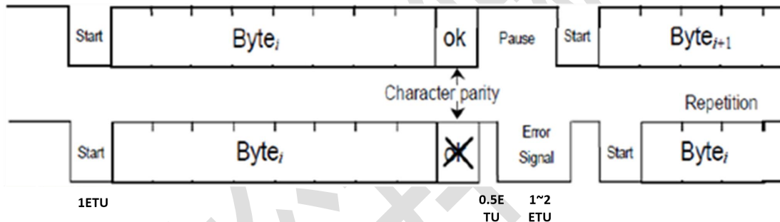
图 20-8: ISO7816 接口时序
