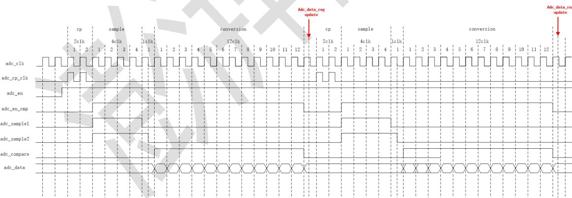
图 23-2 连续转换时序
