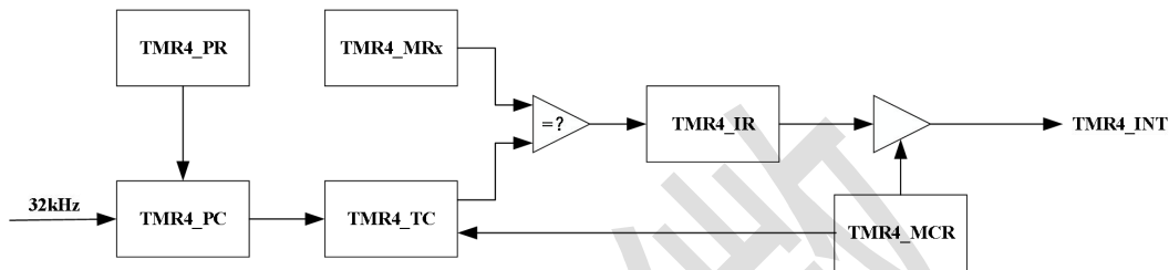
图 14-1 低功耗定时器工作原理图
