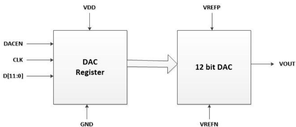
图 24-1 DAC 功能框图
