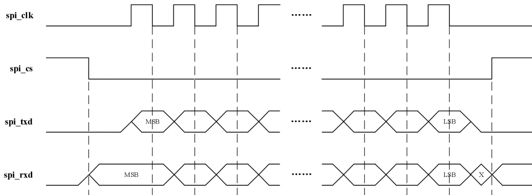
图 21-6: 模式 10 时序图 (SCLKP=10)
