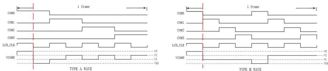
图 16-2 2-COM 模式下，Type A，Type B 驱动波形示意图
