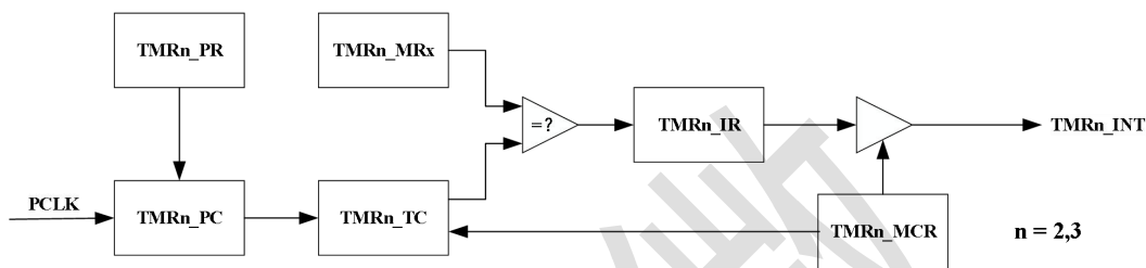
图 13-1 定时器 TMR2 工作原理图
