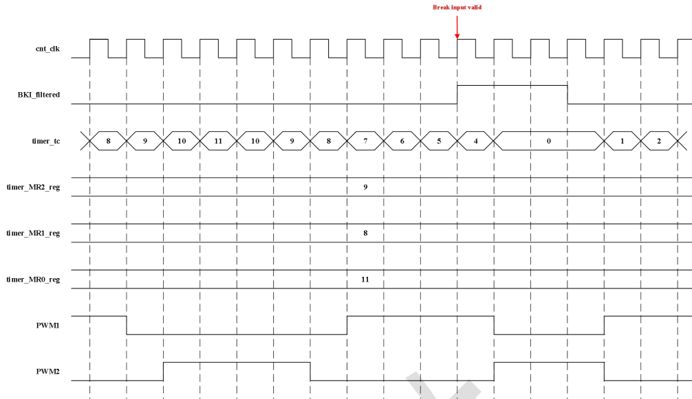
图 10-24 刹车输入有效电平时，独立 PWM 输出波形
