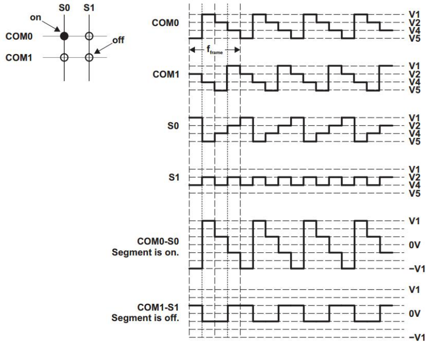
图 16-3 2-COM 模式下，1/3 偏压下的 TypeA 波形
