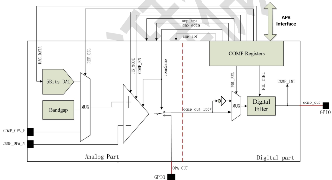
图25-1 比较器结构框图
