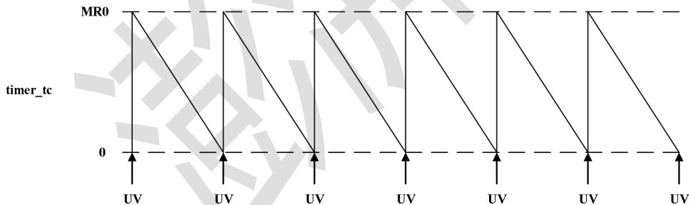
图 14-2 递减计数示意图
