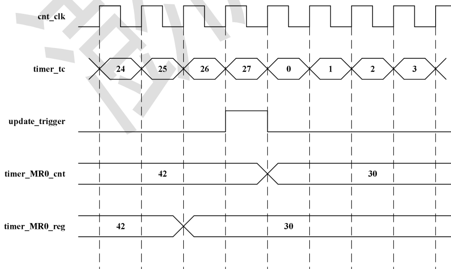
图 12-10 递增计数时手动更新匹配值
