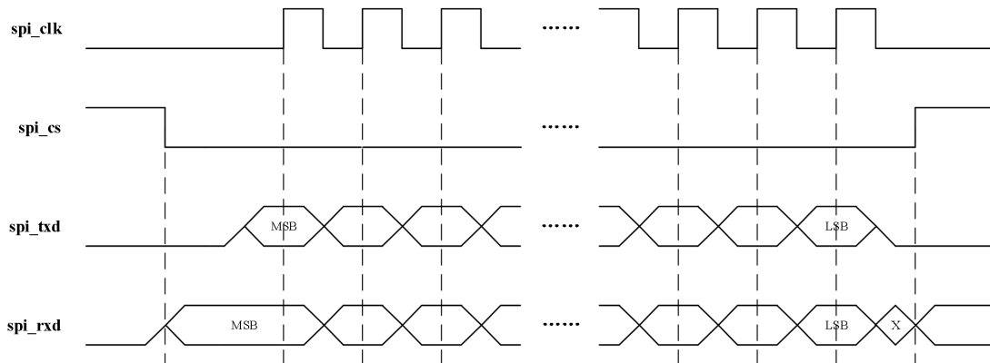
图 21-4 模式 00 时序图 (SCLKP=00)
