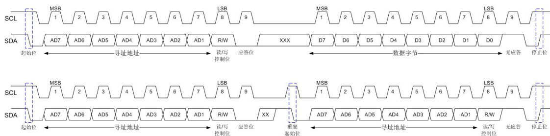
图22-1 I 2 C总线通讯波形示意图
