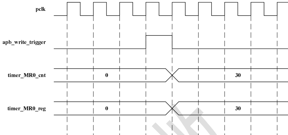
图 12-6 定时器未使能时匹配值更新
