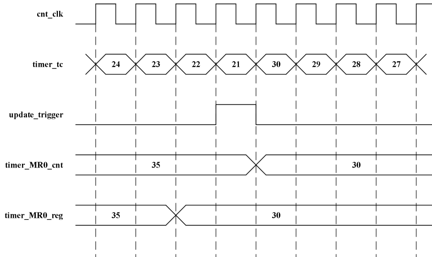
图 12-11 递减计数时手动更新匹配值
